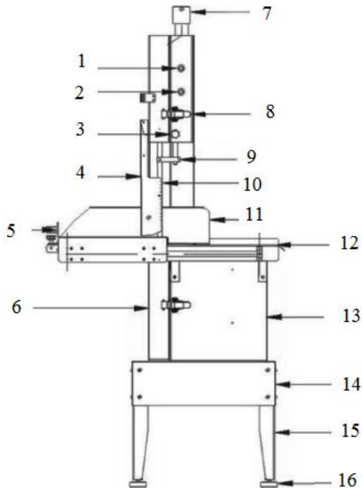
Рис. 1 Общий вид оборудования (для модели FA-400А, эскиз может отличаться от представленного, но основные элементы остаются неизменными).
